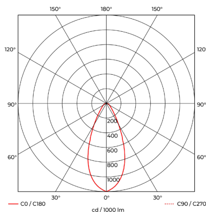
HH240LED4060
