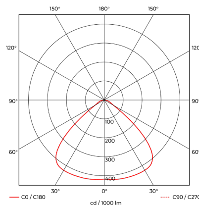
HH240LED40120
